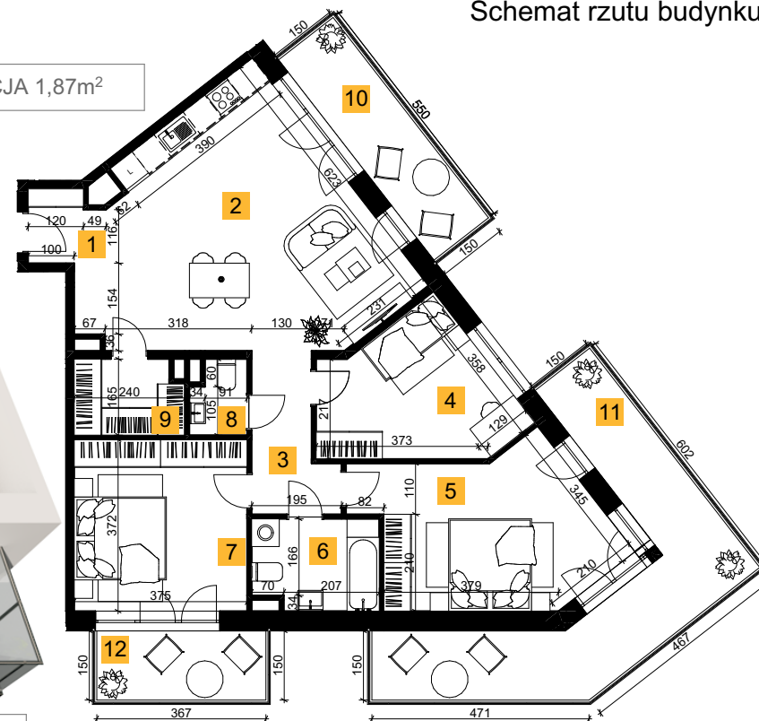
Rzut lokalu
