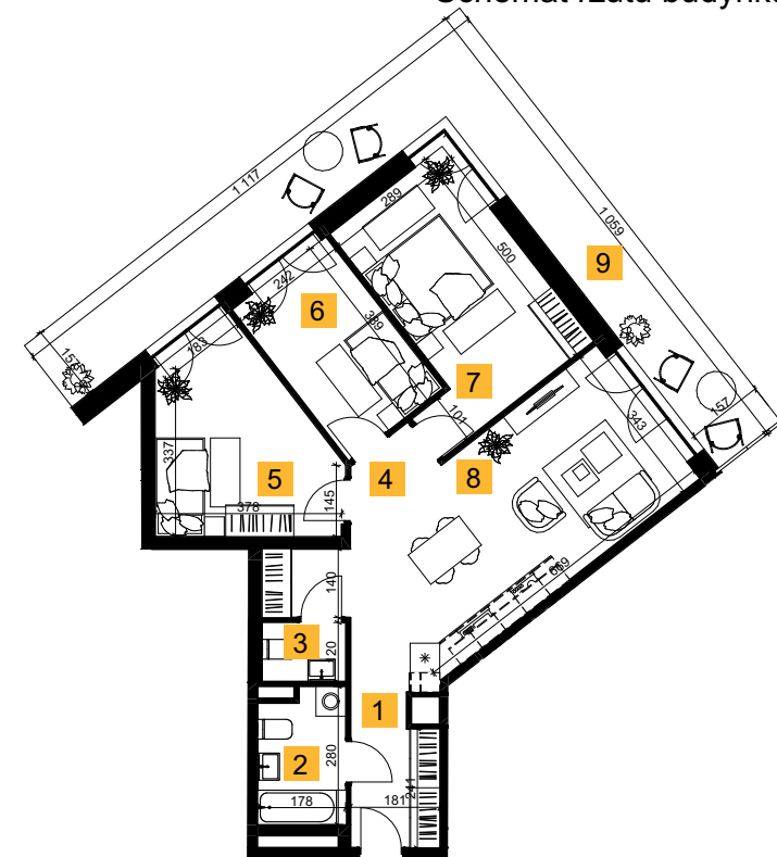
Rzut lokalu
