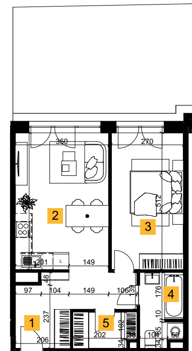
Rzut lokalu
