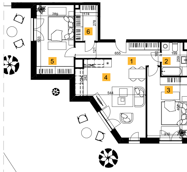
Rzut lokalu
