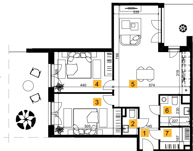
Rzut lokalu
