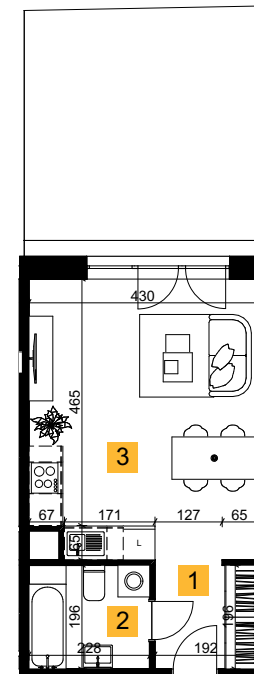
Rzut lokalu
