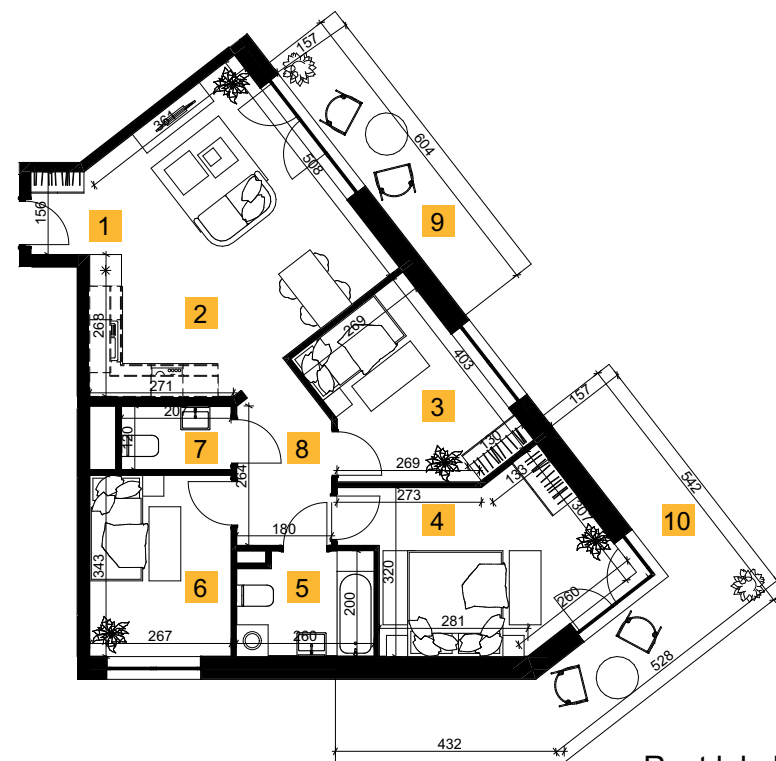
Rzut lokalu
