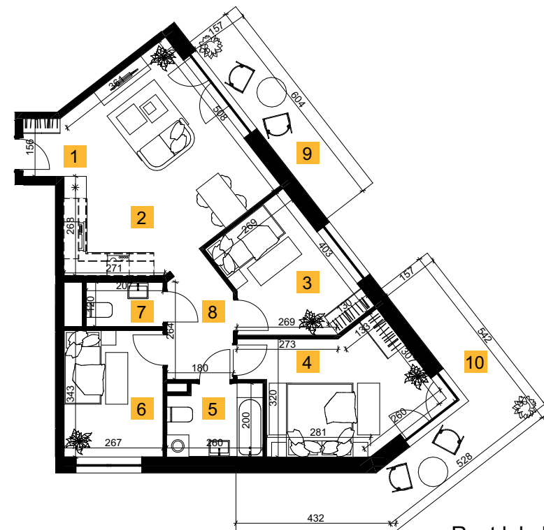
Rzut lokalu
