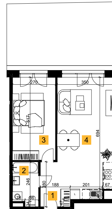
Rzut lokalu
